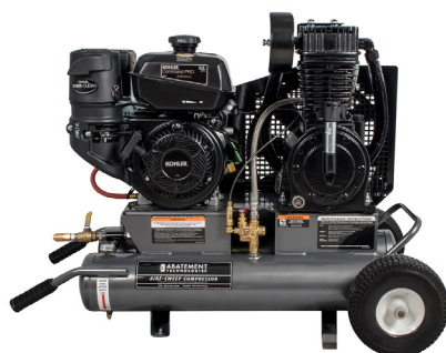
NUMÉRO DE PIÈCE: C17GK - ENSEMBLE DE COMPRESSEUR TOUT INCLUS
