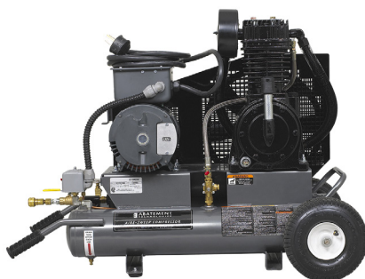
NUMÉRO DE PIÈCE: C17E - ENSEMBLE DE COMPRESSEUR TOUT INCLUS
